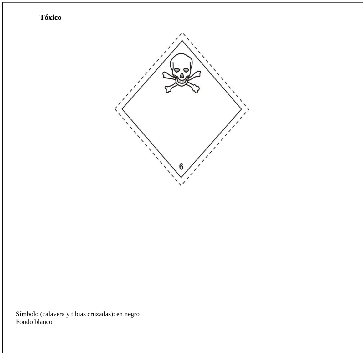
Figura 6.14. Sustancia tóxica, Clase 6, División 6.1
