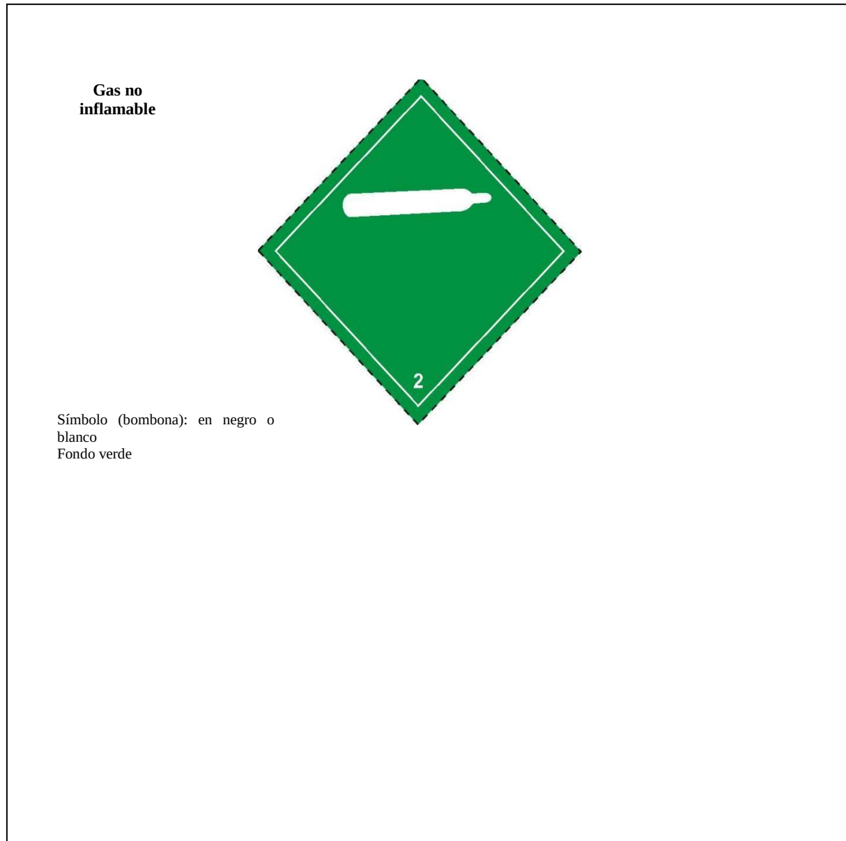
Figura 6.6. Gas no inflamable, no tóxico, Clase 2, División 2.2
