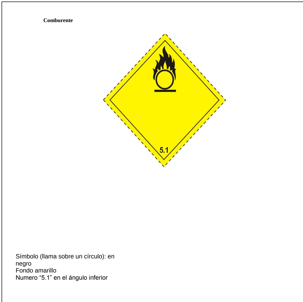
Figura 6.12. Sustancia comburente, Clase 5
