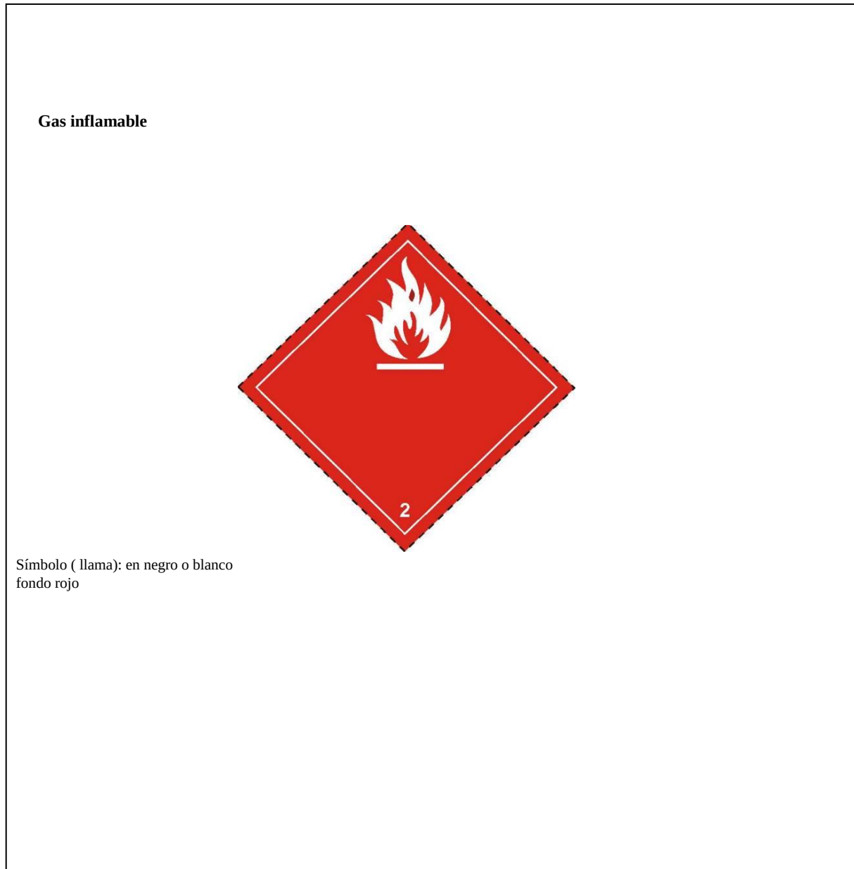
Figura 6.5. Gas inflamable, Clase 2, División 2.1
